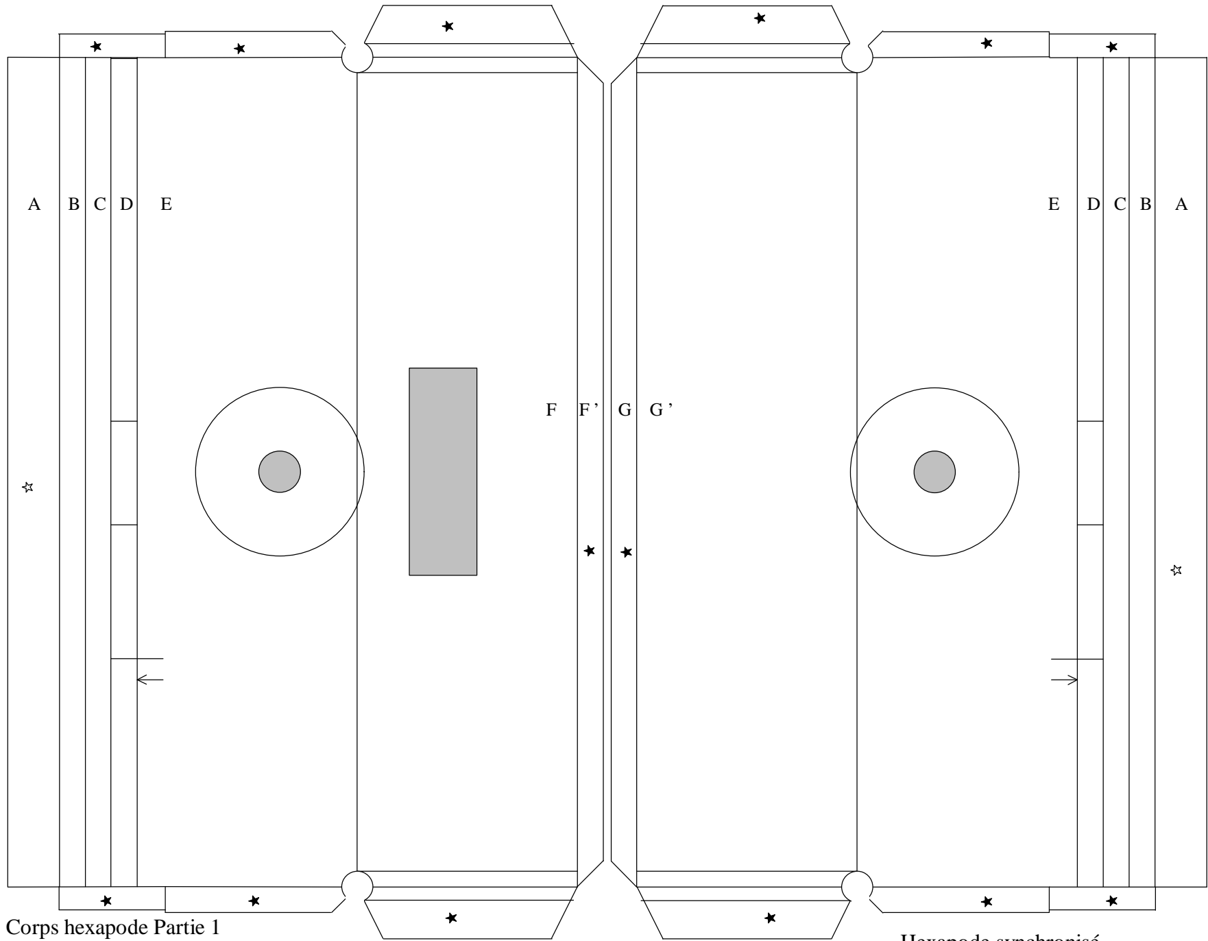
Hexapode synchronisé
